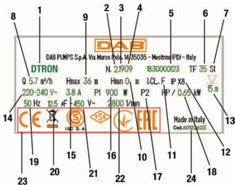
Rys. 4 Tabliczka znamionowa
